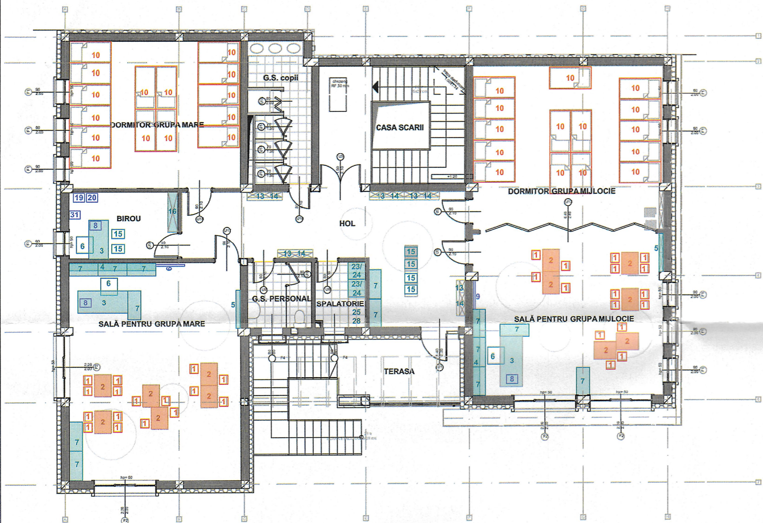
PLAN ETAJ
